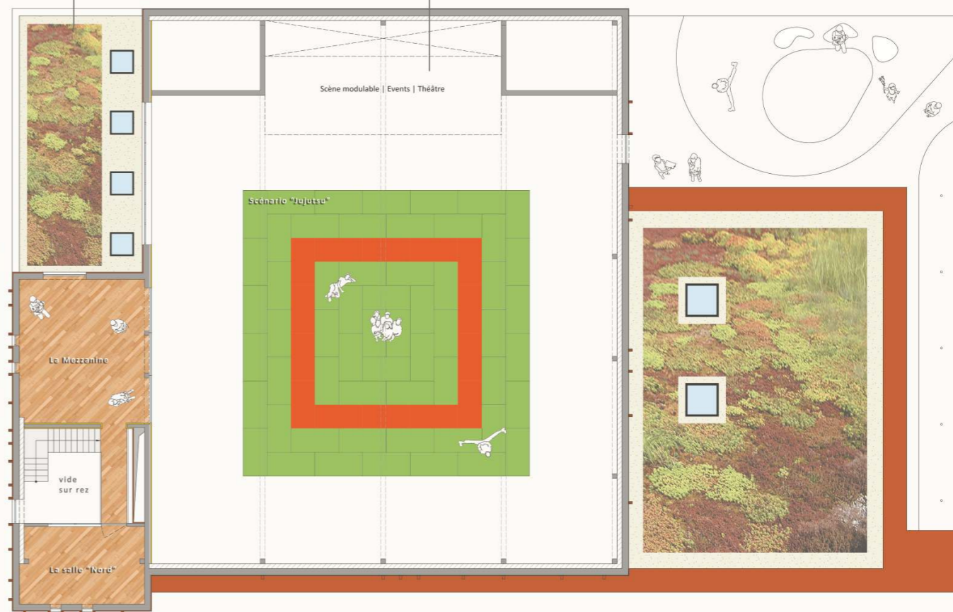
Vue en plan REZ+1 Ech. 1/100
